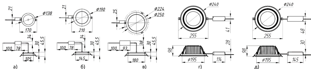
Рисунок 1 — Габаритные чертежи: а) Сейлинг 10Вт, б) Сейлинг 20Вт, в) Сейлинг 30Вт, г) Сейлинг 40Вт, д) Сейлинг 60Вт.
