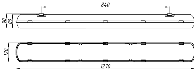
Рисунок 1 – Габаритные размеры светильника ЛСП 2x36.
