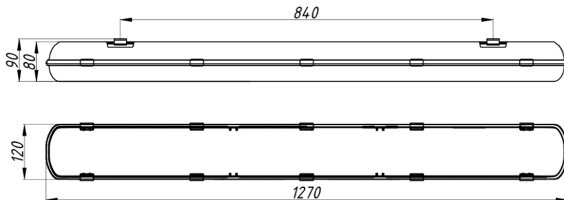
Рисунок 1 – Габаритные размеры светильника ЛСП 2х36.
